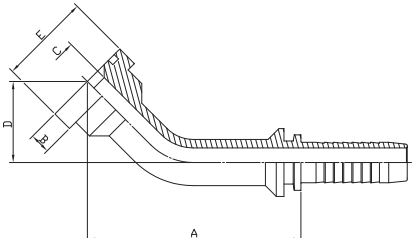
FLANGE SUPERCAT 45° ELBOW:PASC4
