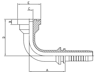
FLANGE SUPERCAT 90° ELBOW:PASC9
