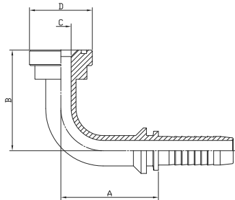
FLANGE 90° ELBOW KOMATSU:PAJK9
